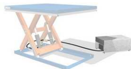
Külön álló motor fém védőburkolattal
